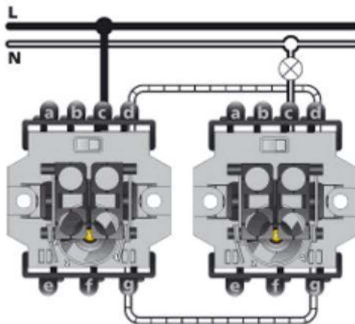
Wechselschaltung Two-way switching
