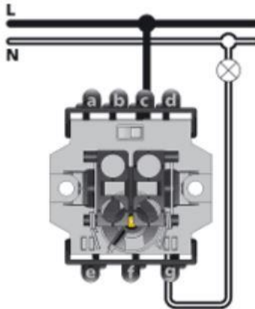
Ausschaltung One-way switching
